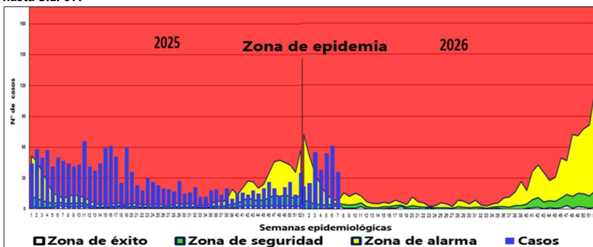
Figura N° 06. Canal endémico de casos de dengue en la Provincia de Alto Amazonas – 2025-2026 hasta S.E. 07.
