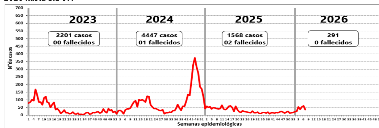
Figura N° 05. Tendencia semanal de casos de dengue en la Provincia de Alto Amazonas, 2023-2026 hasta S.E 07.
