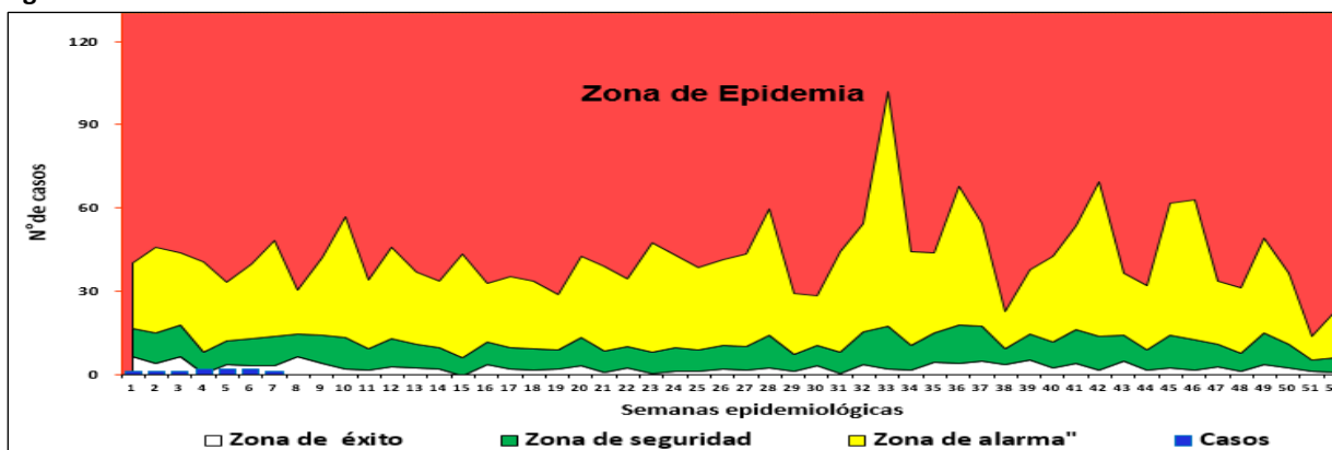
Figura N° 01. Canal de casos de malaria en la Provincia de Alto Amazonas – 2026 a la S.E. 07.
